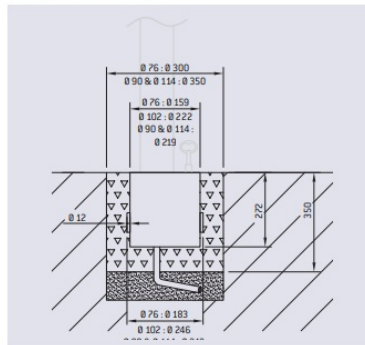
PLAN DE SCÉLLEMENT
