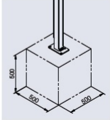
PLAN DE SCELLEMENT
